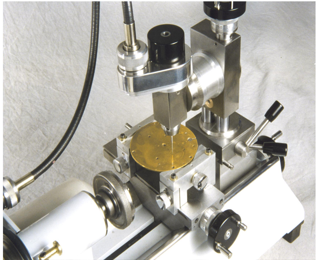
Alesatura dei fori ovalizzati dall'usura su platine varie
