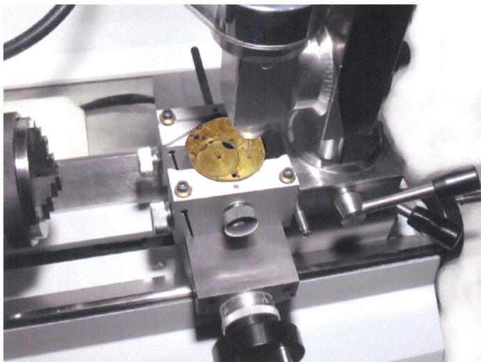
Centratura micrometrica al foro originale
